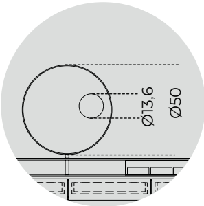
Specchio ingranditore
